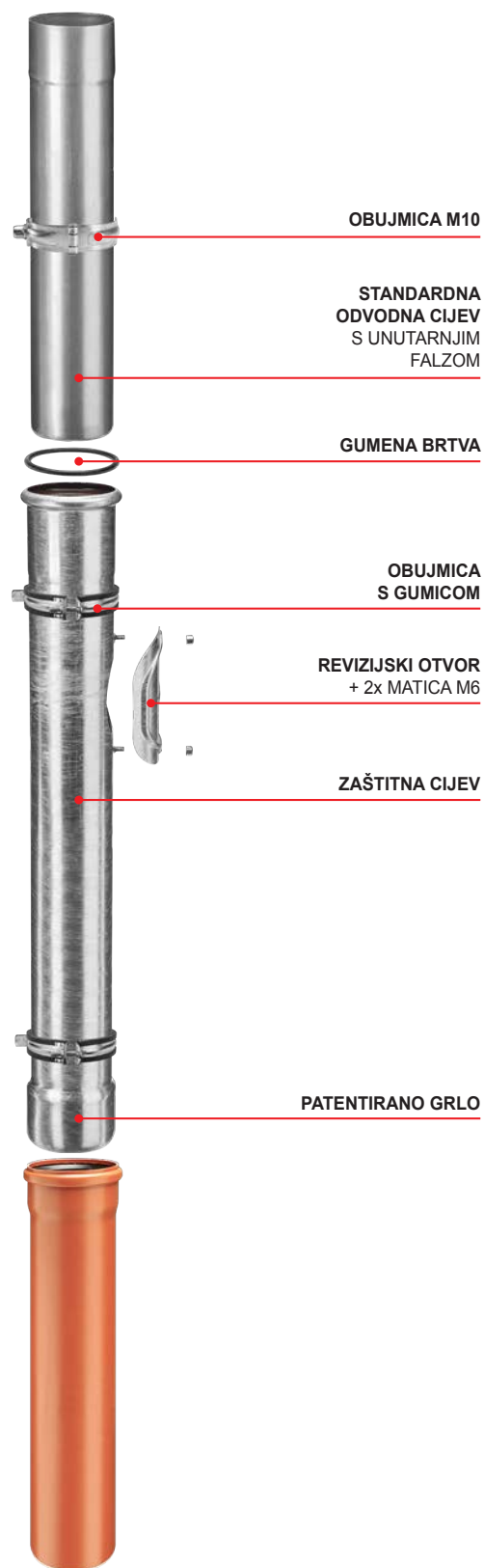
VERZIJA B PVC KANALIZACIJSKA CIJEV
