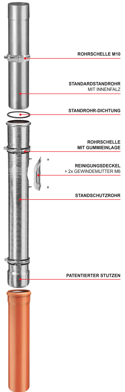
VARIANTE B KANALISATIONSROHR PVC
